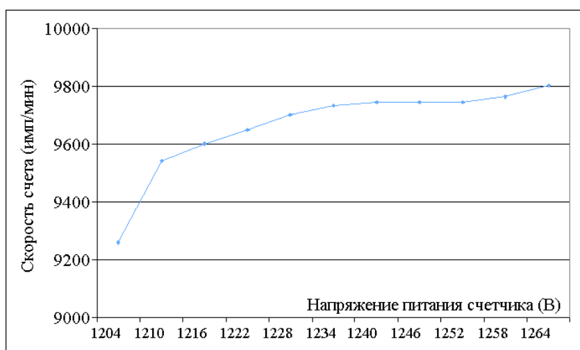
Рис.11. Плато счетной характеристики от напряжения питания счетчика СММ 67Э.
