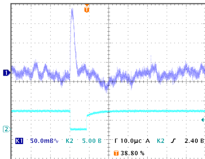
Рис.6. Вид полезного сигнала на фоне «короны» счетчика СММ 67 (счетчик «советского» периода).
