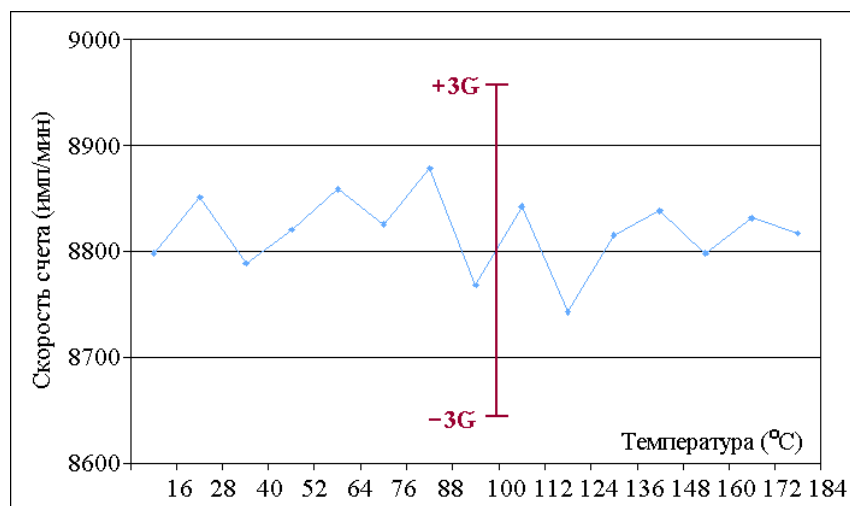
Рис.12. Изменение скорости счета счетчика СНМ 67Э при изменении температуры окружающей среды.
