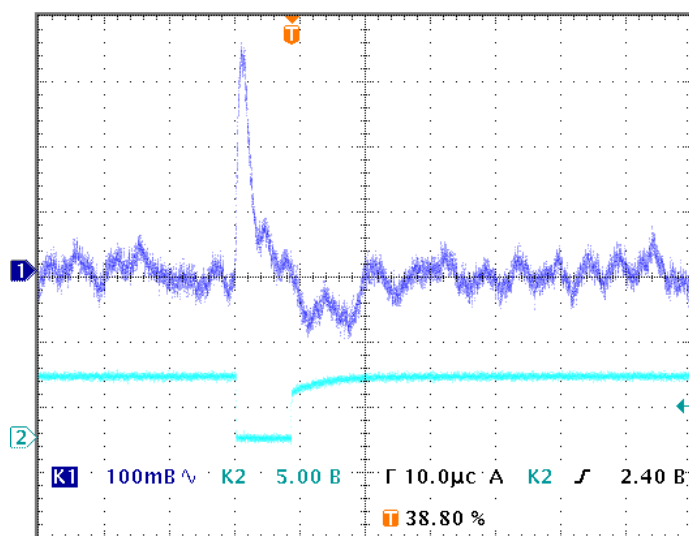
Рис.7. Вид полезного сигнала на фоне «короны» счетчика СММ 67Э (счетчик производства ЭХП).
