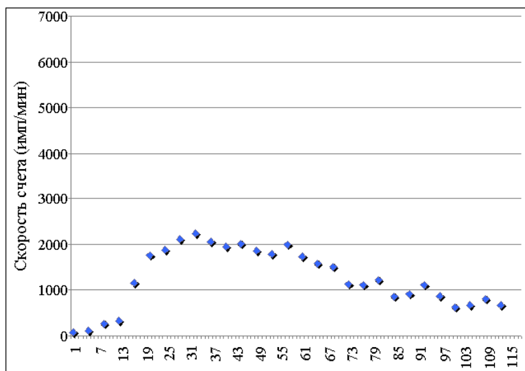
Рис. 10. Дифференциальный спектр сигналов со счетчика СММ 67Э, включенного в режиме пропорционального счета.
